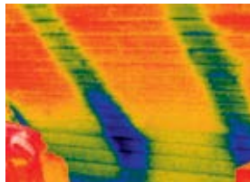
hőhidas tető
